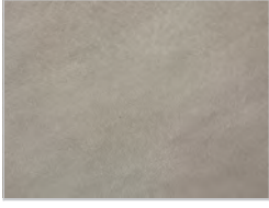
pelle camoscio: 28
